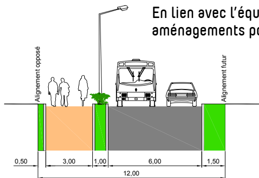
Profil des aménagements qui seront réalisés rue du Douanier Rousseau et Chemin de la Lande.
